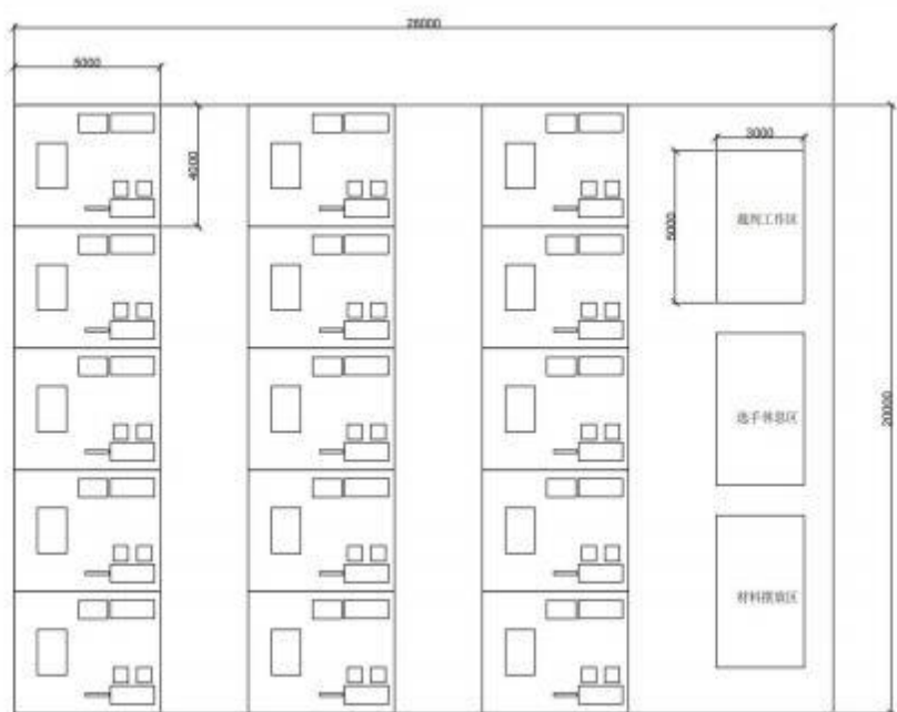
图 1 场地布局示意图
